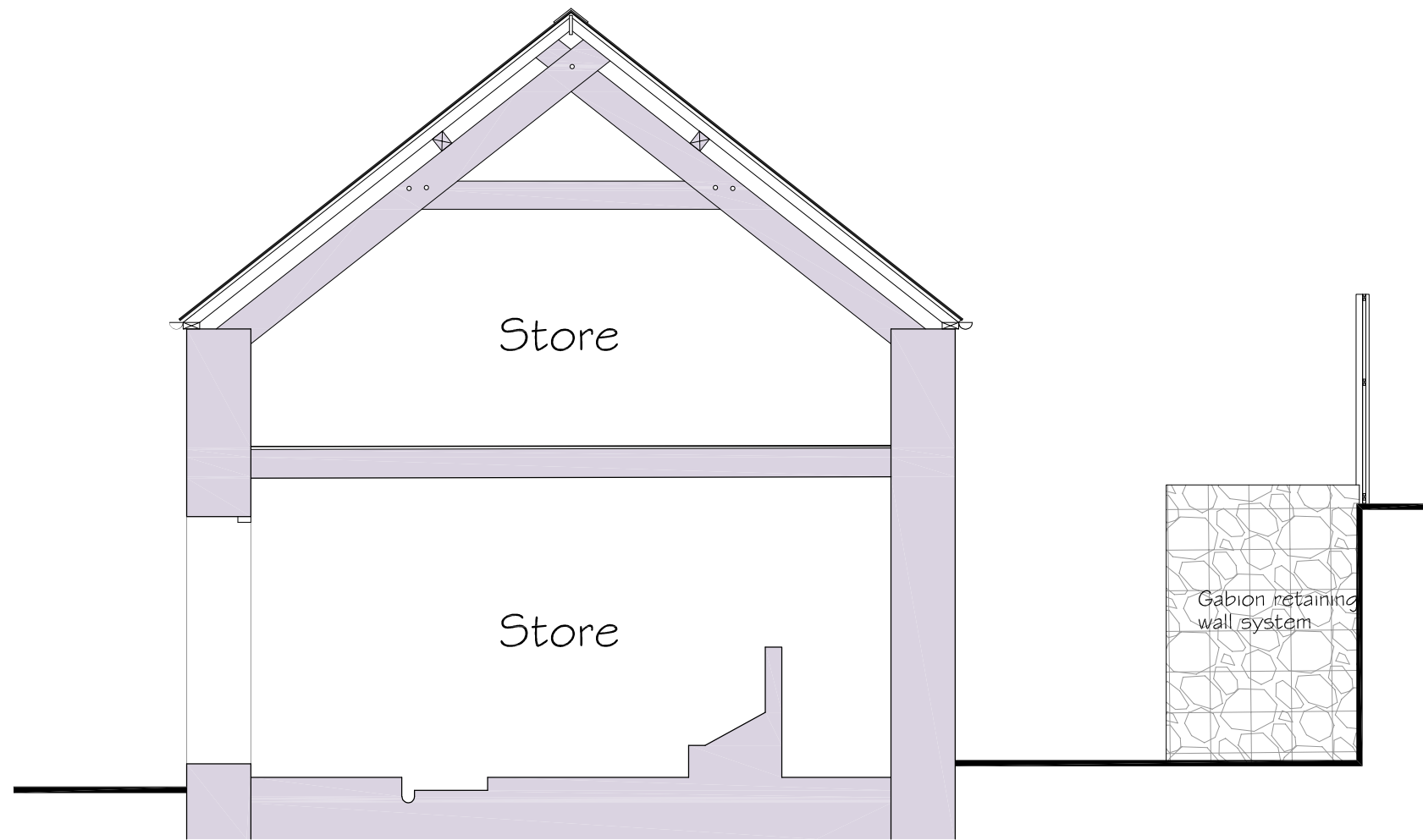
Section A-A 1:50
